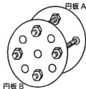
組立図 5
